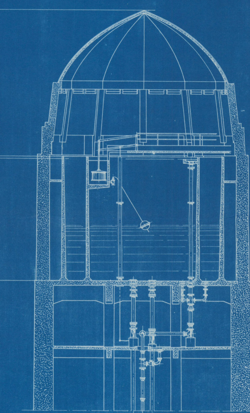
DOORSNEDE D-Q
