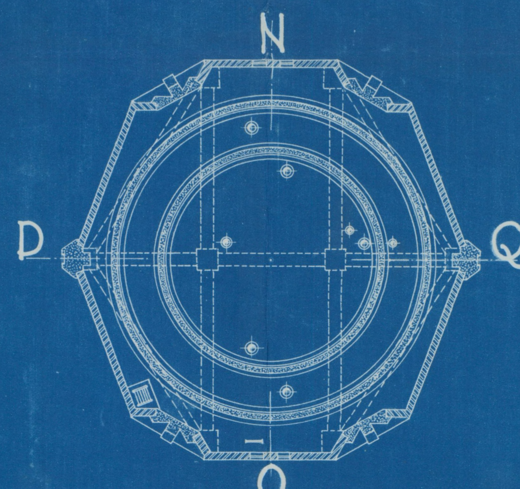
DOORSNEDE J-K
