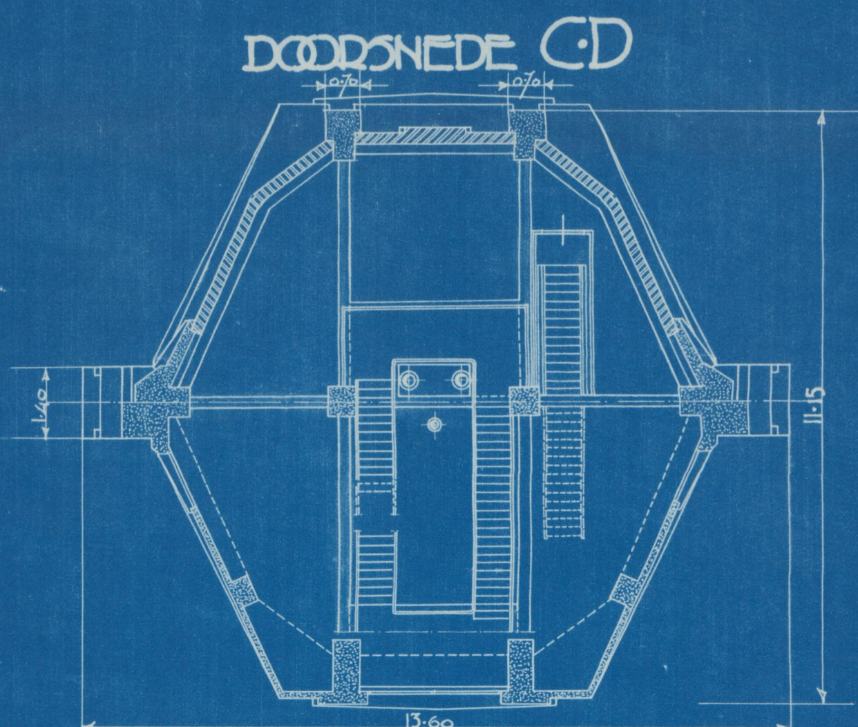
DOORSNEDE A-B
