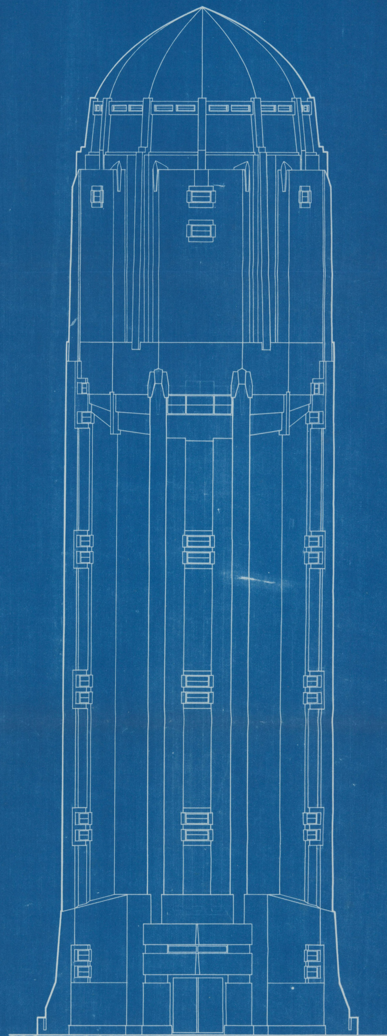
VORSTAANZICHT
