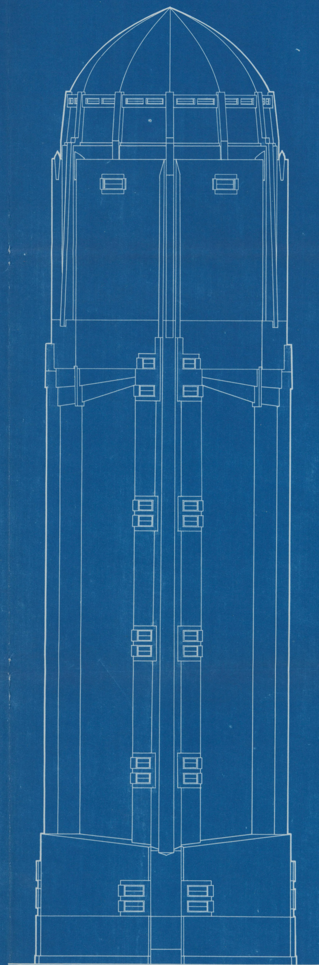
ZIJVAANZICHT
