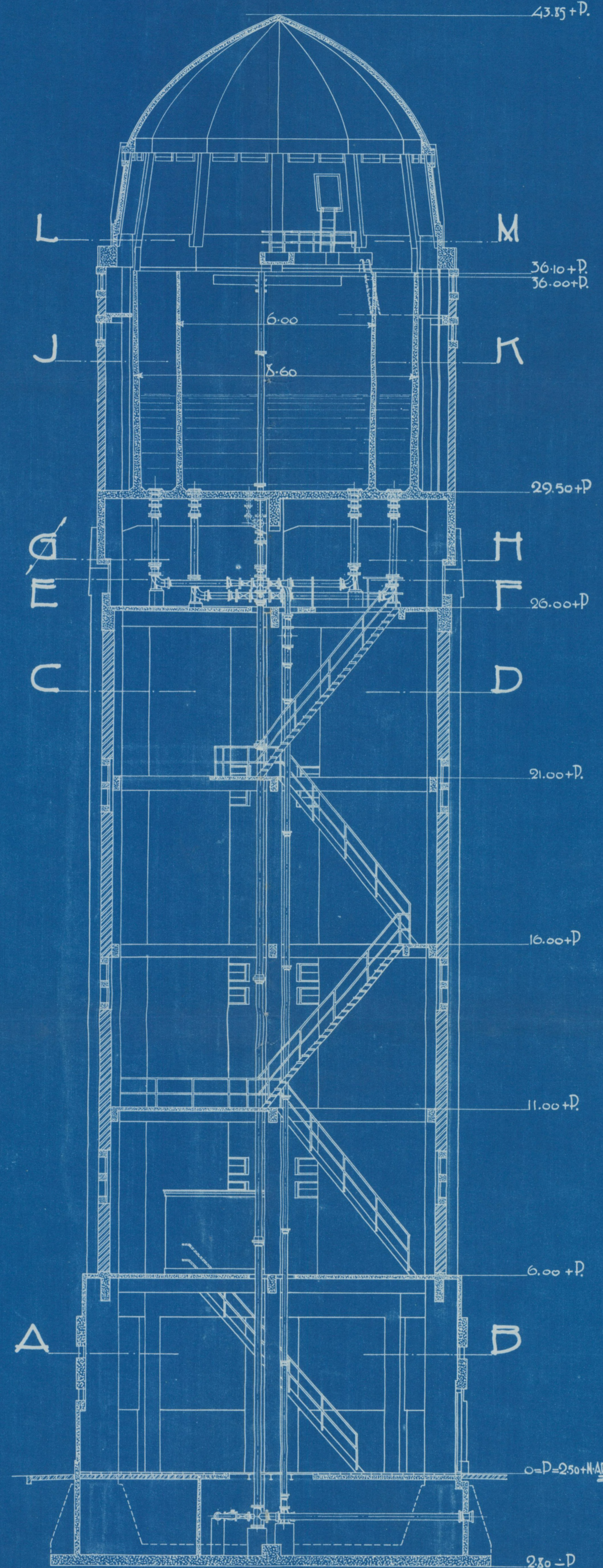
DOORSNEDE N-O
